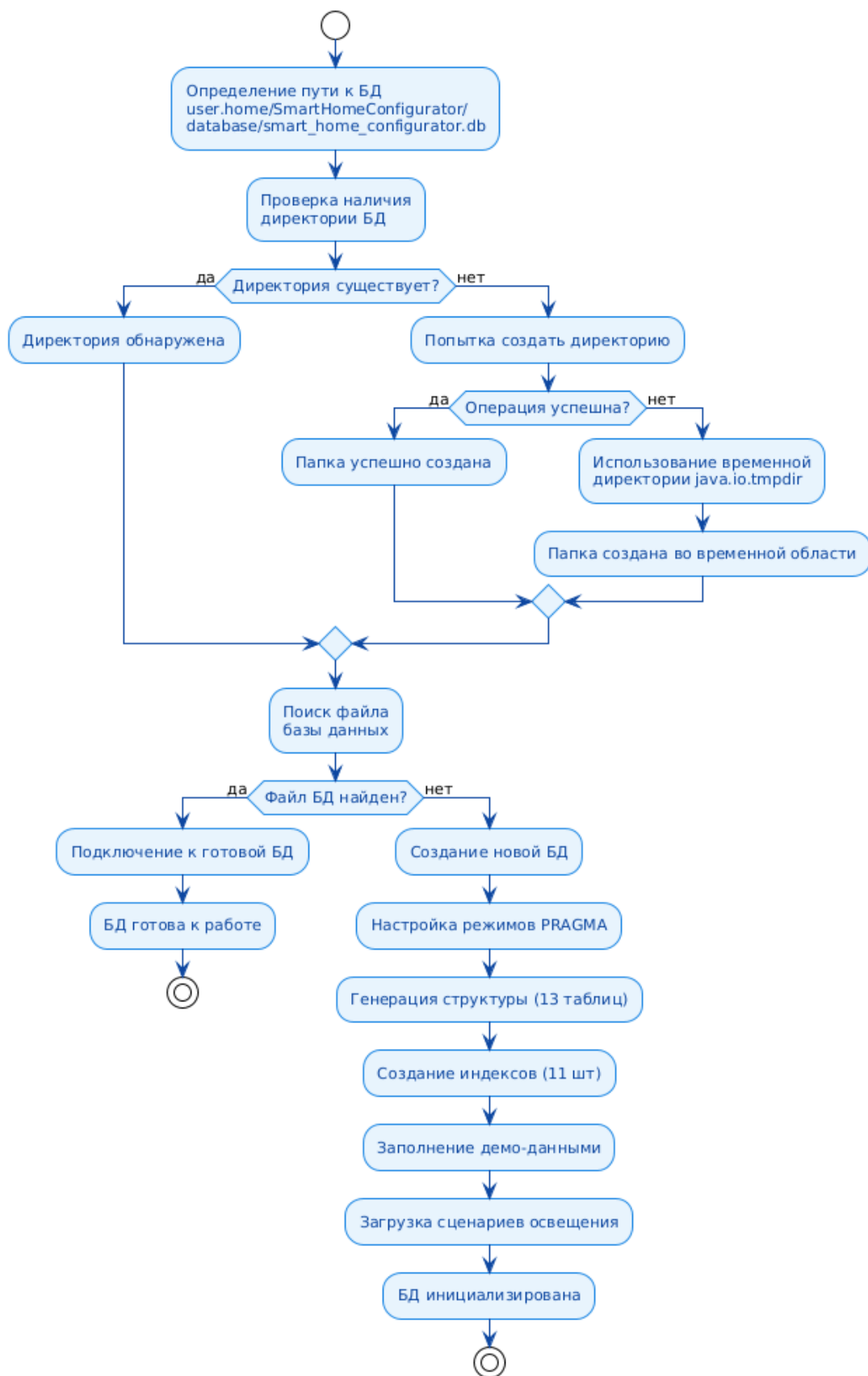
Рисунок 8 – Алгоритм инициализации базы данных
