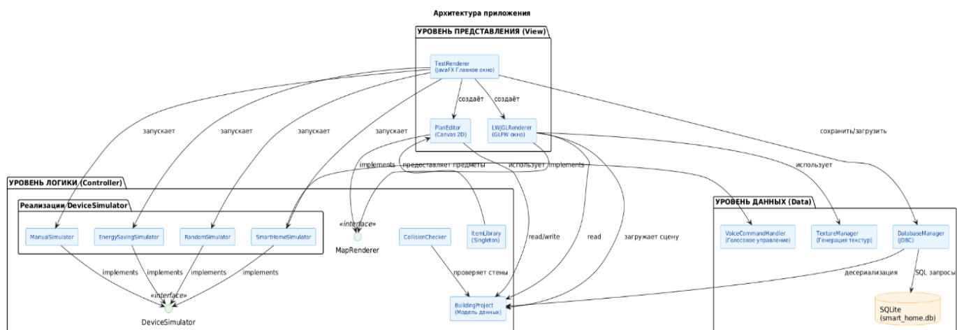
Рисунок 3 – Архитектура приложения
